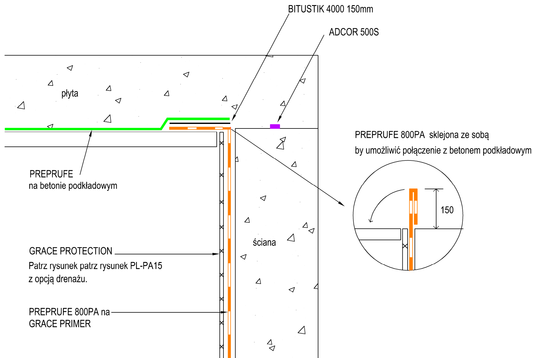
DETAL POŁĄCZENIA ŚCIANY W GÓRNYM POZIOME PŁYTY SEKCJA
